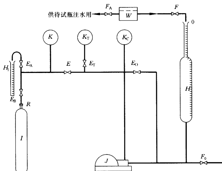
W—试验用水水槽;J—水泵;I—专用瓶;R—专用接头;F、F 0 、F A —低压阀;H—量管(固定安置,“0”刻度线位于上端);K C —压力测量仪表(指示、控制泵出口压力用);K—压力测量仪表(读取试验压力用);K T —精密压力表(校验其他压力测量仪表用);E、E O 、E A 、E T —高压阀(E、E O 为等容积阀,E T 试验时关闭);H 1 —滴定管
