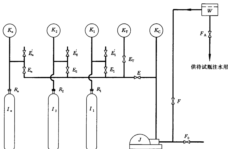
W—试验用水水槽； K_C —压力测量仪表（指示、控制泵出口压力用）； K_1 \sim K_n —压力测量仪表（读取试验压力用）； I_1 \sim I_n —受试瓶； E, E_T, E_1 \sim E_n, E'_1 \sim E'_n —高压阀（试验时 E_T 关闭）； K_T —精密压力表（检验其他压力测量仪表用）； J —水压泵； R_1 \sim R_n —专用接头； F, F_0, F_A —低压阀
