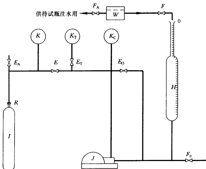
W—试验用水水槽; J—水压泵; I—受试瓶; R—专用接头; F、F 0 、F A —低压阀; H—量管(固定安置,“0”刻度线位于上端); K C —压力测量仪表(指示、控制泵出口压力用); K—压力测量仪表(读取试验压力用); K T —精密压力表(校验其他压力测量仪表用); E、E O 、E A 、E T —高压阀(E、E O 为等容积阀, E T 试验时关闭)
